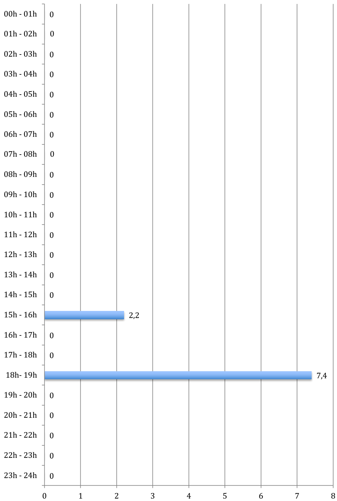
Cantidades de lluvia registradas por horas en BÉTERA "SUD" (Torre en Conill) el 25/09/21 (en l/m²)
