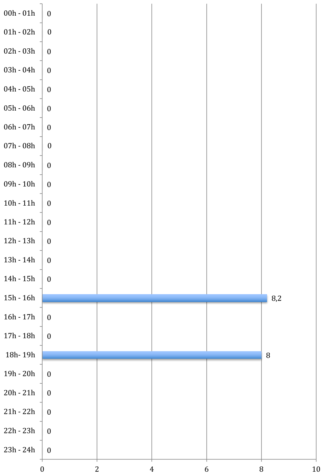
Cantidades de lluvia registradas por horas en BÉTERA "CENTRO" (núcleo urbano) el 25/09/21 (en l/m²)
