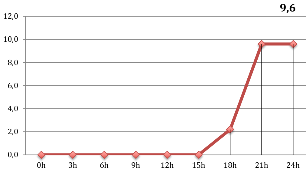
Evolución lluvia acumulada en BÉTERA "SUD" (Torre en Conill) el 25/09/21 en períodos de 3 horas (en l/m 2 )
