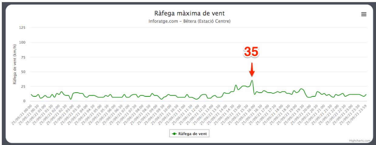
Ráfagas de viento registradas en BÉTERA "CENTRO" (núcleo urbano) el 18/09/21 (en km/h)
