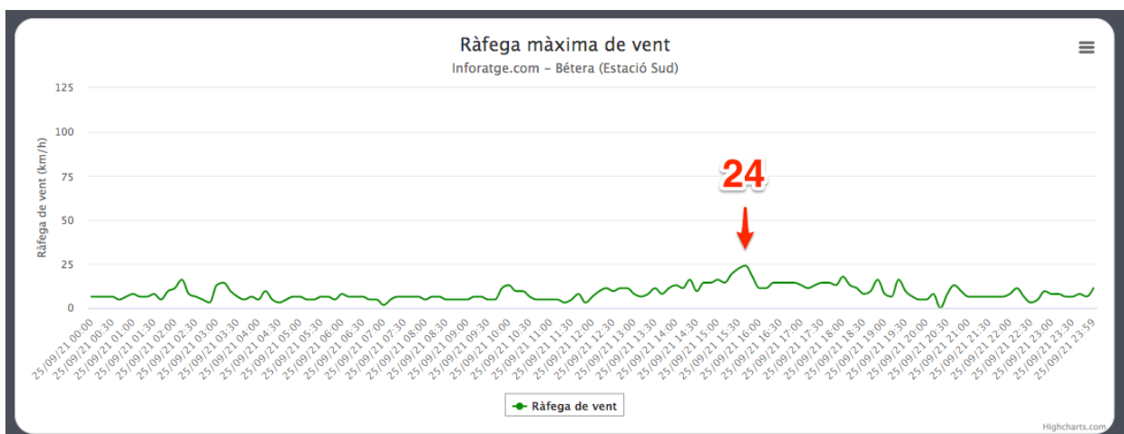
Ráfagas de viento registradas en BÉTERA "SUD" (Torre en Conill) el 25/09/21 (en km/h)
